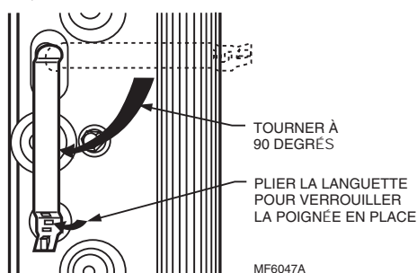
Fig. 8. Installer les poignées au bout de la cellule qui est la plus près de la porte d'accès.
